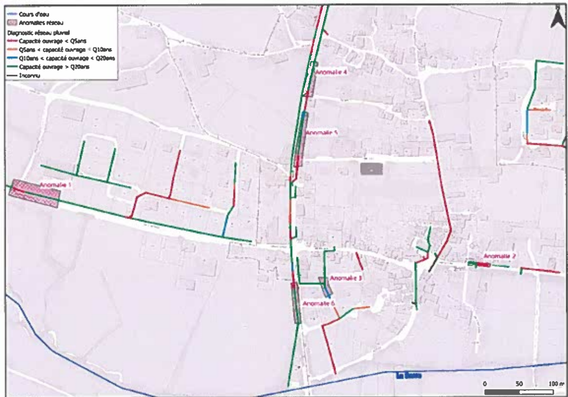
Figure 44 : Anomalies de section du réseau d'eaux pluviales et diagnostic
